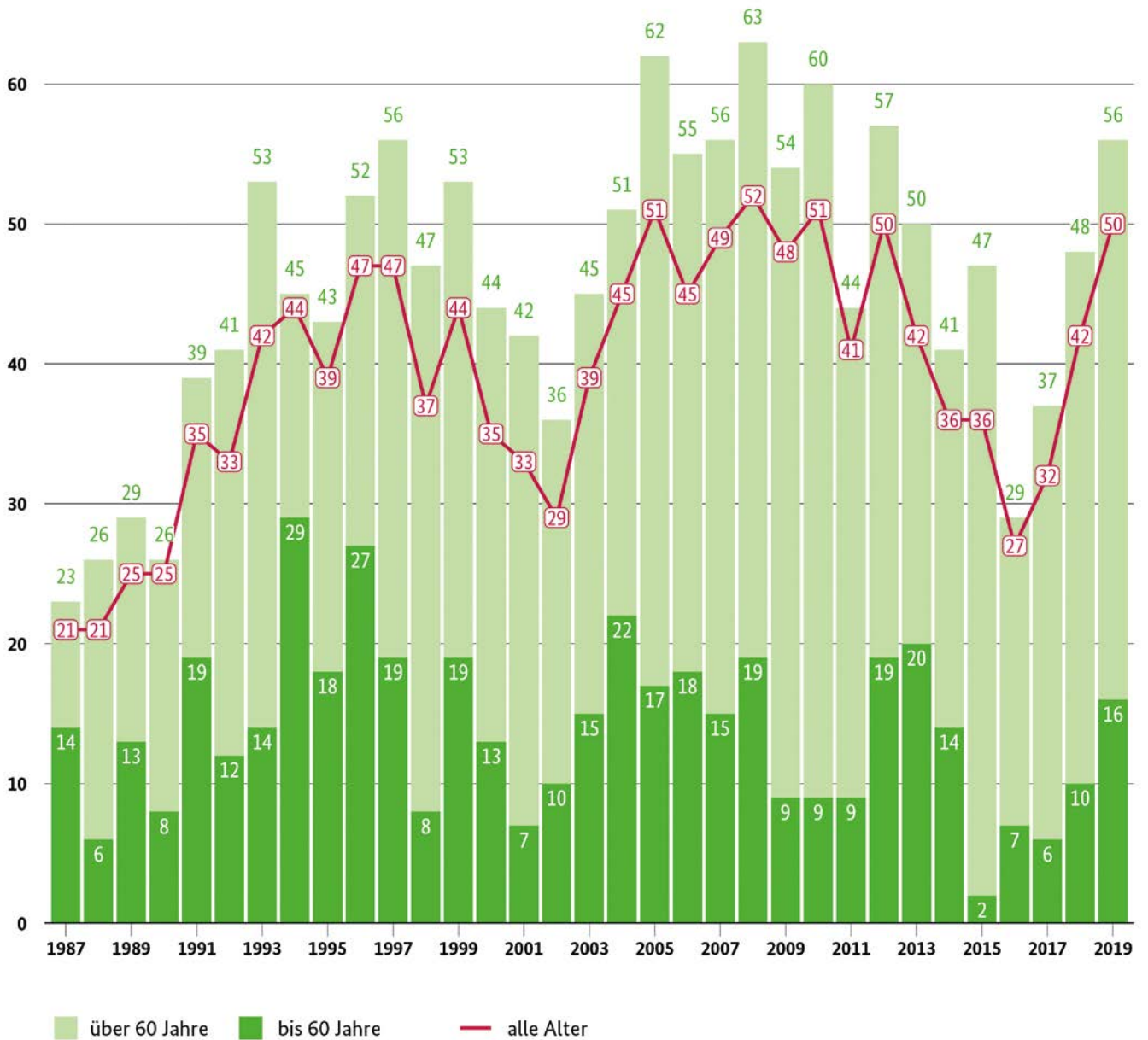
Abbildung 21: Eiche – Anteil der deutlichen Kronenverlichtungen nach Altersgruppen und insgesamt (in Prozent)
