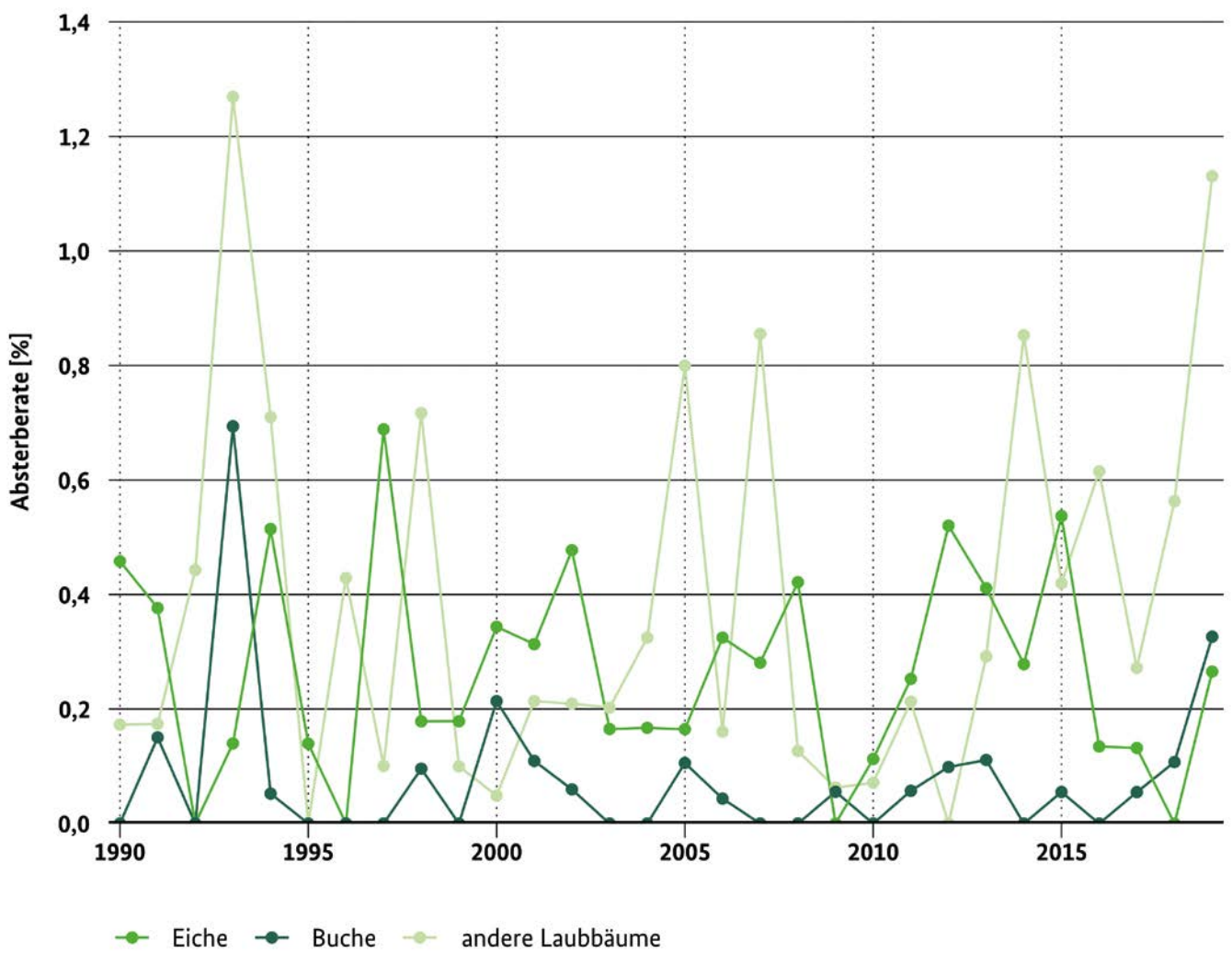
Abbildung 25: Absterberaten bei den Laubbäumen
