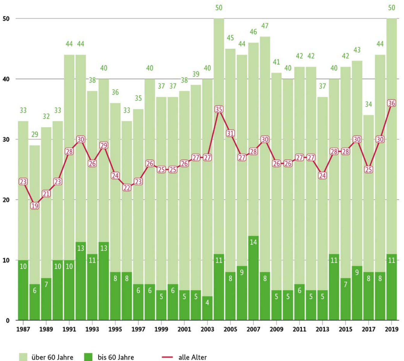
Abbildung 17: Fichte – Anteil der deutlichen Kronenverlichtungen nach Altersgruppen und insgesamt (in Prozent)
