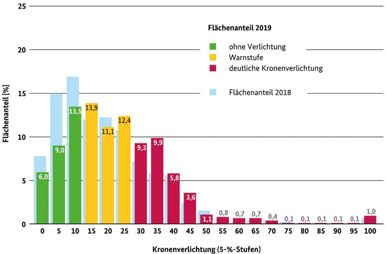
Abbildung 9: Andere Nadelbäume – Häufigkeitsverteilung der 5-%-Stufen der Kronenverlichtung 2018 und 2019
