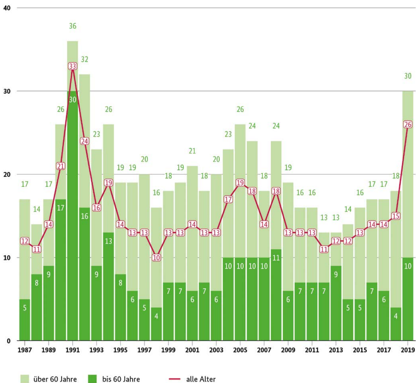
Abbildung 18: Kiefer – Anteil der deutlichen Kronenverlichtungen nach Altersgruppen und insgesamt (in Prozent)
