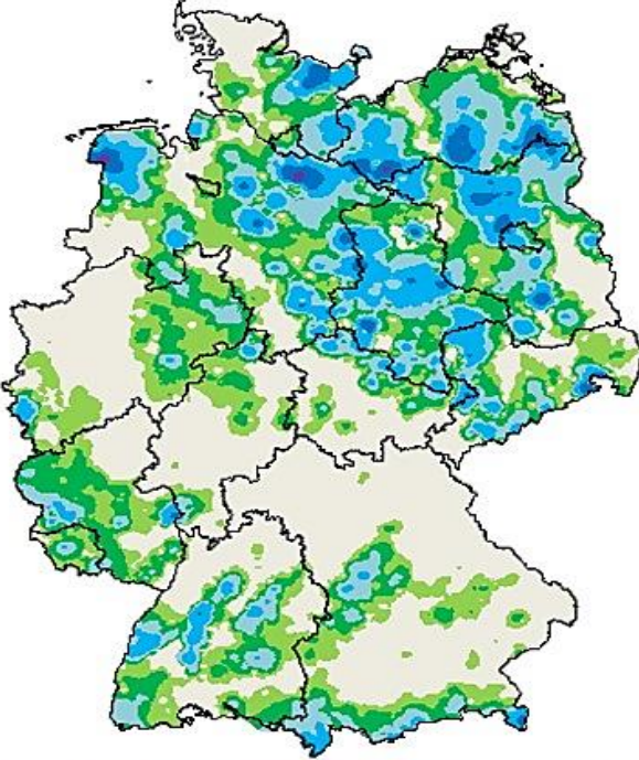
Niederschlag (Tagessumme) Mo 15.08.2022
