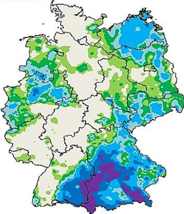
Niederschlag (Tagessumme) Fr 19.08.2022
