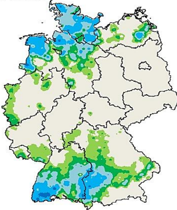
Niederschlag (Tagessumme) Mi 17.08.2022
