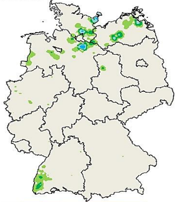
Niederschlag (Tagessumme) Di 16.08.2022
