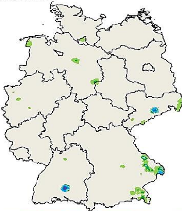
Niederschlag (Tagessumme) So 21.08.2022
