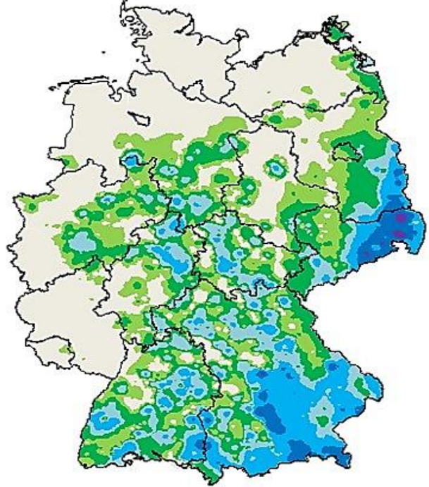
Niederschlag (Tagessumme) Sa 20.08.2022
