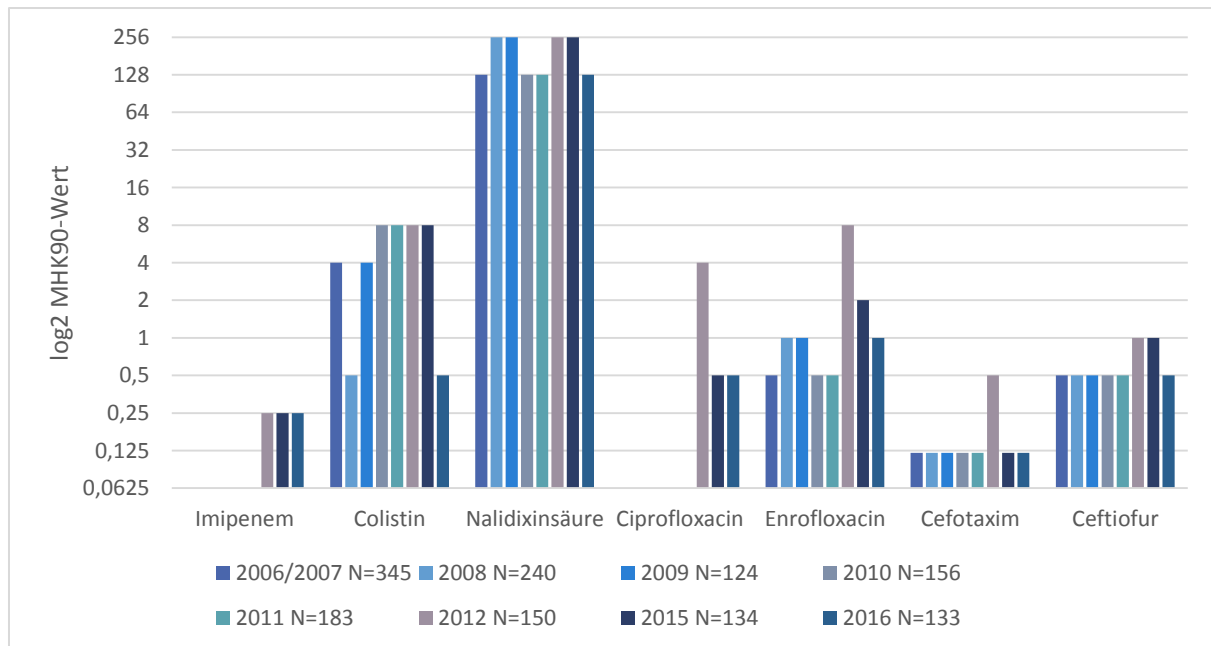
Abbildung 12: Vergleich der MHK_{90} -Daten gegenüber antimikrobiellen Substanzen von E. coli , isoliert aus erkrankten Ferkeln (Untersuchungszeitraum 2006/2007-2016, Ciprofloxacin und Imipenem ab 2012 untersucht)
