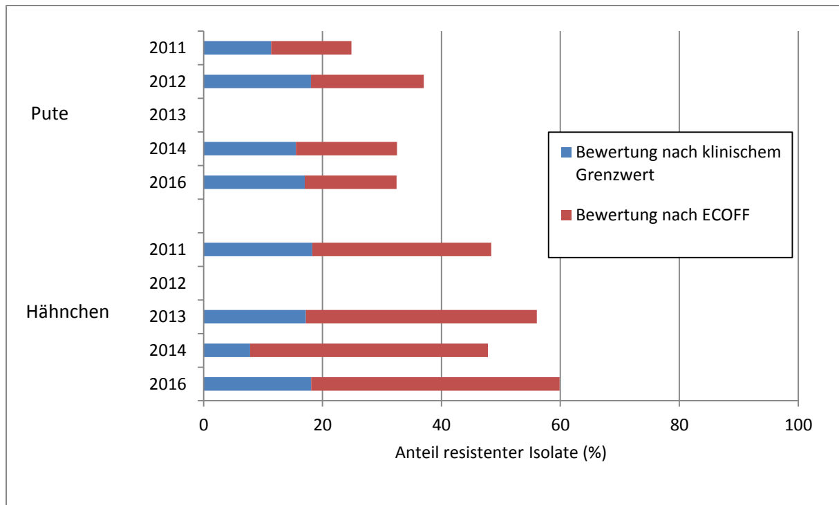
Abbildung 22: Anteil Ciprofloxacin-resistenter E. coli Isolate beim Geflügel 2011-2016 mit minimaler Hemmkonzentration über 0,06mg/l (ECOFF) bzw. 0,5 mg/l (klinischer Breakpoint nach EUCAST). Isolate aus dem Jahr 2011 stammten aus den Beständen, die Daten der anderen Jahre aus Proben von Blinddarminhalt am Schlachthof.
