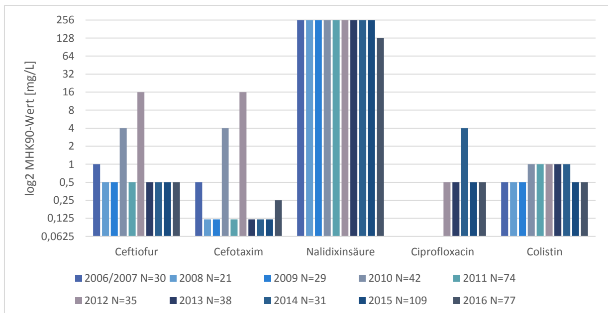
Abbildung 5: Vergleich der MHK 90 -Daten gegenüber antimikrobiellen Substanzen von E. coli , isoliert aus erkrankten Masthähnchen (Untersuchungszeitraum 2006/2007-2016, Ciprofloxacin und Imipenem erst ab 2012 untersucht)
