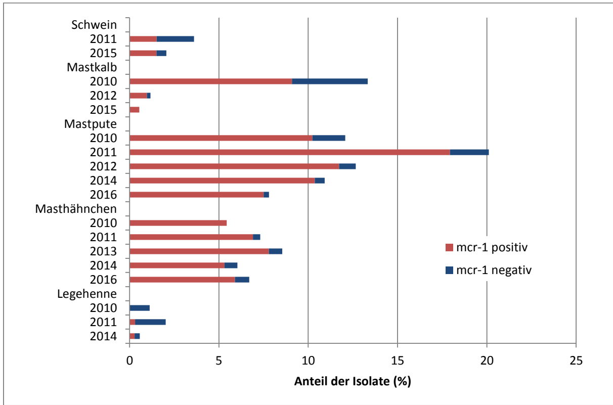
Abbildung 24: Colistin-Resistenz von E. coli von Tieren aus dem Zoonosen-Monitoring mit (rot) und ohne (blau) mcr-1 Gen (Irrgang et al 2016, aktualisiert für 2016)
