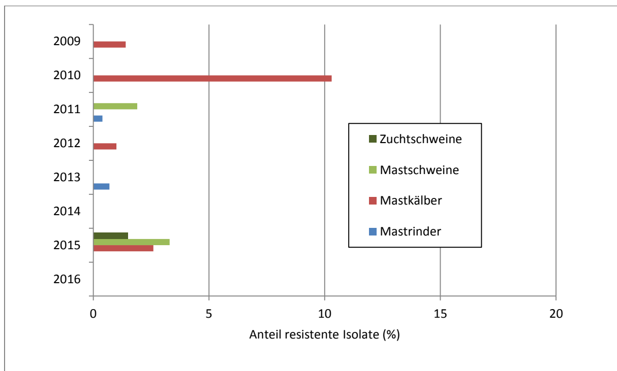
Abbildung 18: Anteil Cephalosporin-resistenter E. coli aus nicht selektiver Anzucht bei Schweinen und Rindern 2009-2016 (nur untersuchte Jahre dargestellt). Bewertung gemäß Durchführungsbeschluss 2013/652/EU.
