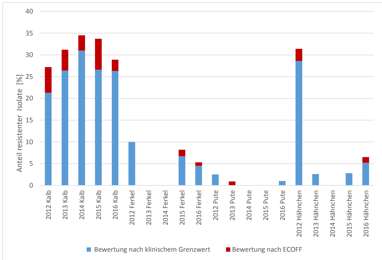
Abbildung 20: Anteil Cefotaxim-resistenter, klinischer E. coli -Isolate bei verschiedenen Tierarten, klinische Isolate 2012-2015 mit minimaler Hemmkonzentration über 0,5 mg/l (ECOFF) bzw. 2 mg/l (klinischer Breakpoint nach EUCAST), Isolate vom Schwein 2013 und 2014 nicht untersucht.
