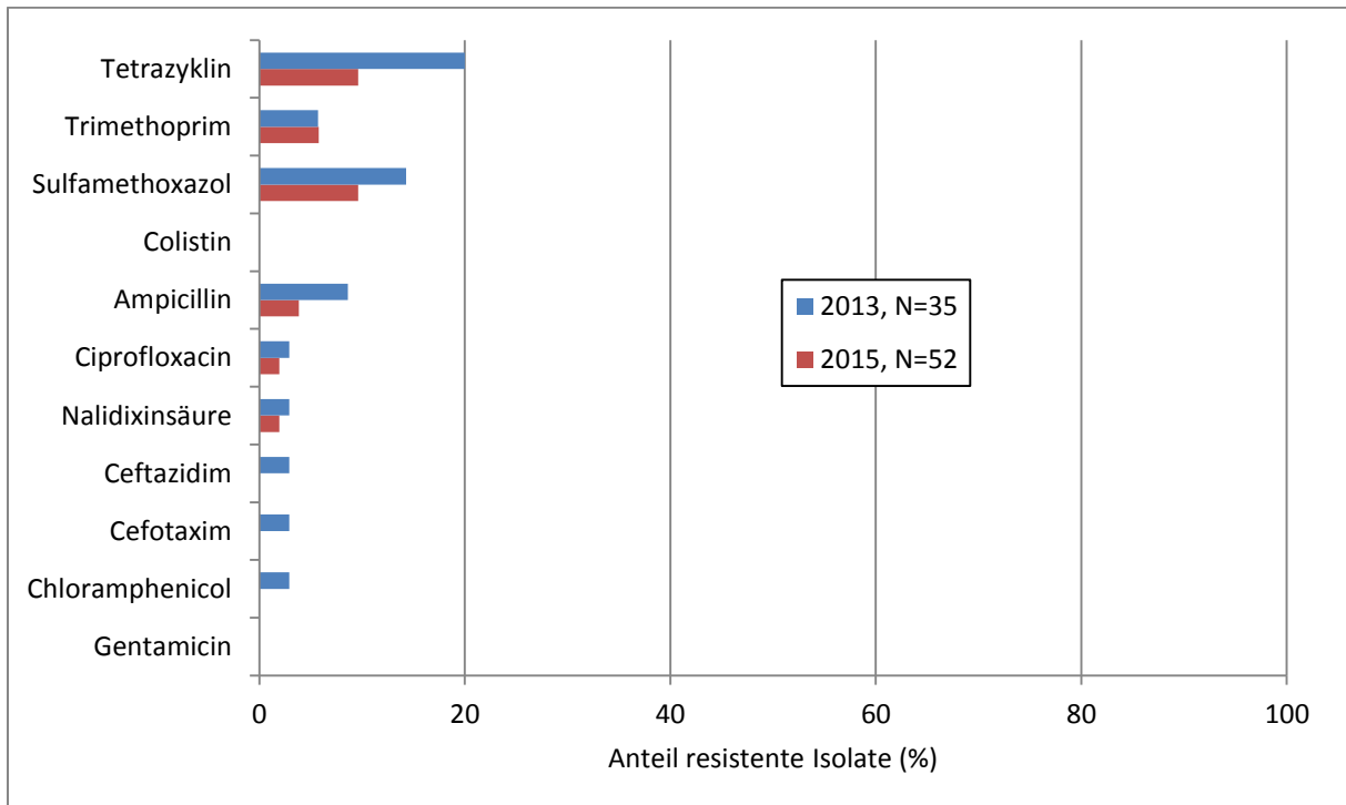
Abbildung 14: Vergleich der Resistenz von E. coli von Rindfleisch aus den Jahren 2013 und 2015 (jeweils Zoonosen-Monitoring). Bewertung gemäß Durchführungsbeschluss 2013/652/EU.
