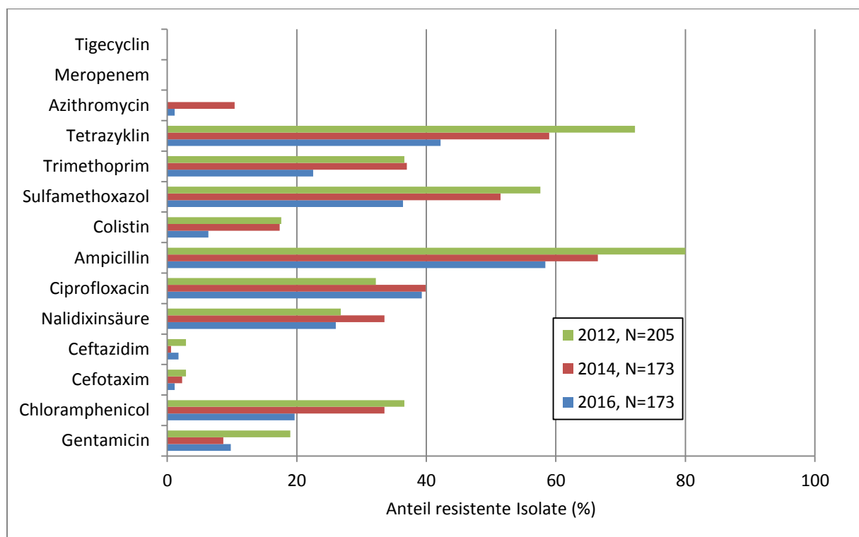
Abbildung 6: Vergleich der Resistenzraten gegenüber antimikrobiellen Substanzen von E. coli aus Mastputenherden aus den Jahren 2012, 2014 und 2016. Tigecyclin, Meropenem und Azithromycin wurden 2012 noch nicht getestet. Bewertung gemäß Durchführungsbeschluss 2013/652/EU.
