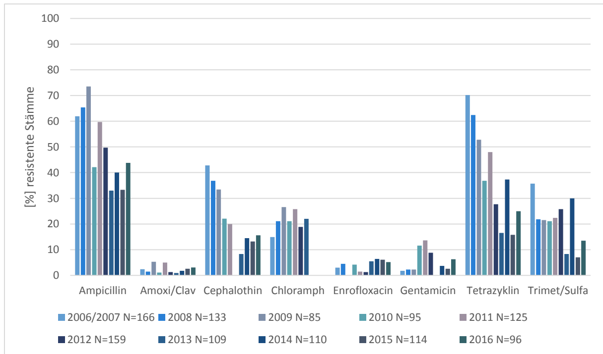
Abbildung 7: Vergleich der Resistenzraten gegenüber antimikrobiellen Substanzen von E. coli isoliert aus erkrankten Puten (Untersuchungszeitraum 2006/2007-2016, Cephalothin 2012 nicht untersucht, Chloramphenicol nur bis 2012 untersucht).
