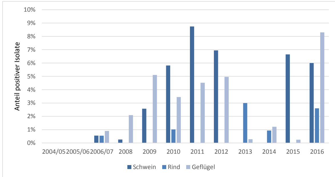
Abbildung 25: Anteil mcr-1 positiver Isolate am gesamten Probeneingang ( E. coli ), Untersuchungszeitraum 2004/2005 bis 2016
