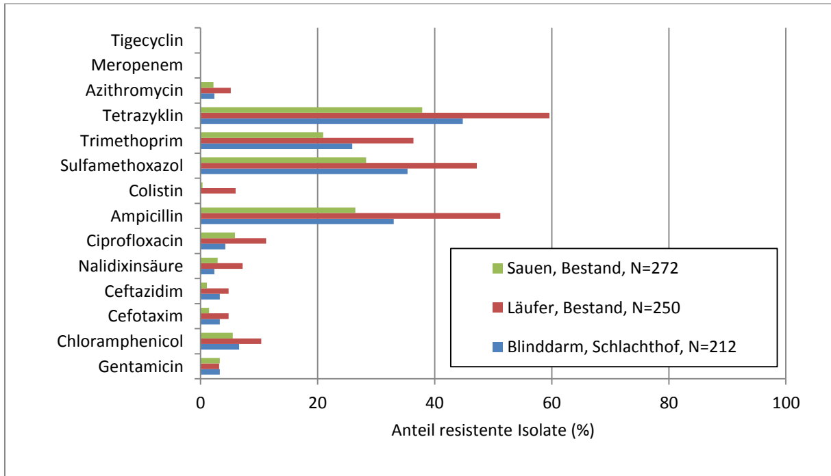
Abbildung 10: Vergleich der Resistenz von E. coli von Sauen, Läufer Schweinen und aus Blinddarmproben von Mastschweinen bei der Schlachtung gegen antimikrobielle Substanzen (Zoonosen-Monitoring 2015). Bewertung gemäß Durchführungsbeschluss 2013/652/EU.
