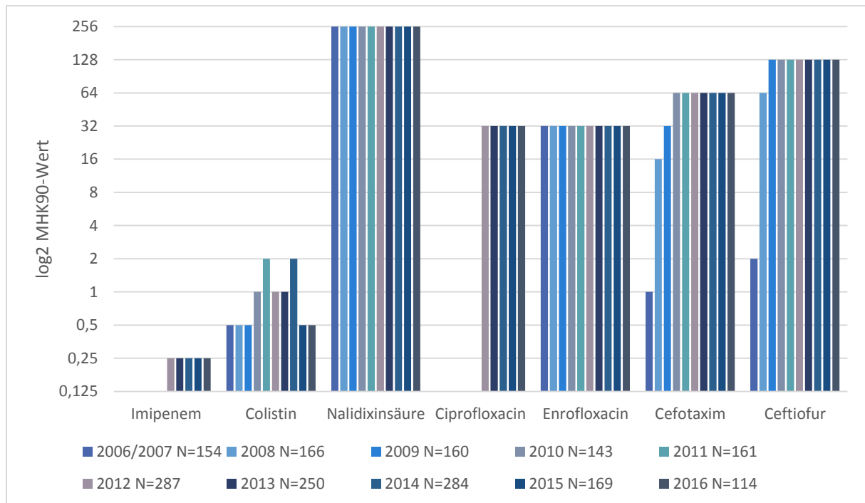
Abbildung 16: Vergleich der MHK_{90} -Daten gegenüber antimikrobiellen Substanzen von E. coli , isoliert aus erkrankten Kälbern (Untersuchungszeitraum 2006/2007-2016, Ciprofloxacin und Imipenem ab 2012 untersucht)
