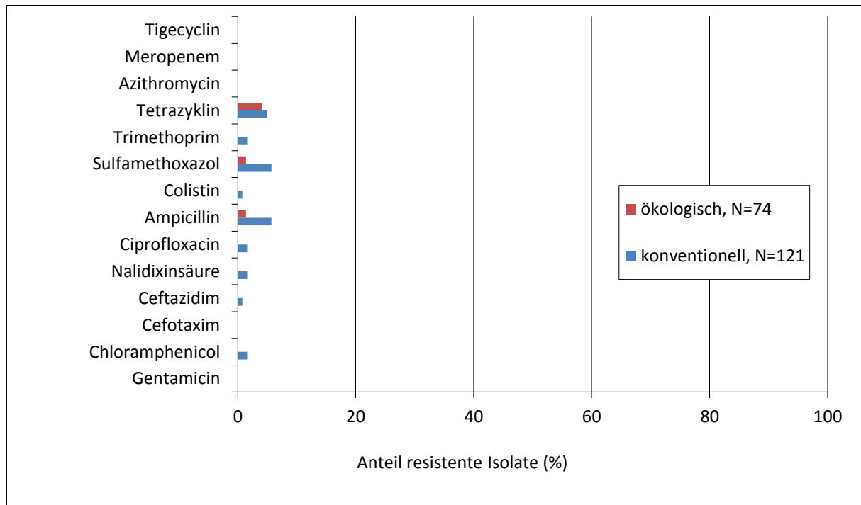
Abbildung 27: Vergleich der Resistenzraten von E. coli aus Tankmilchproben konventioneller und ökologischer Milchviehbetriebe (Zoonosen-Monitoring 2014). Bewertung gemäß Durchführungsbeschluss 2013/652/EU.
