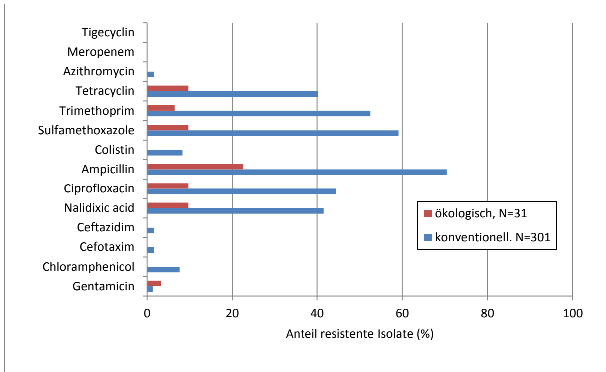
Abbildung 26: Vergleich der Resistenzraten von E. coli aus konventionellen und ökologischen Masthähnchenherden, Zoonosen-Monitoring 2016. Bewertung gemäß Durchführungsbeschluss 2013/652/EU.
