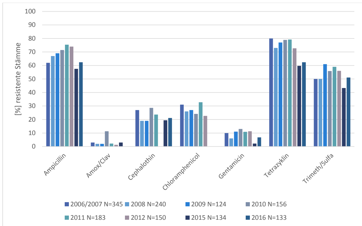
Abbildung 11: Vergleich der Resistenzraten gegenüber antimikrobiellen Substanzen von E. coli isoliert aus erkrankten Ferkeln (Untersuchungszeitraum 2006/2007-2016, 2012 Cephalothin nicht untersucht, Chloramphenicol nur bis 2012 untersucht)
