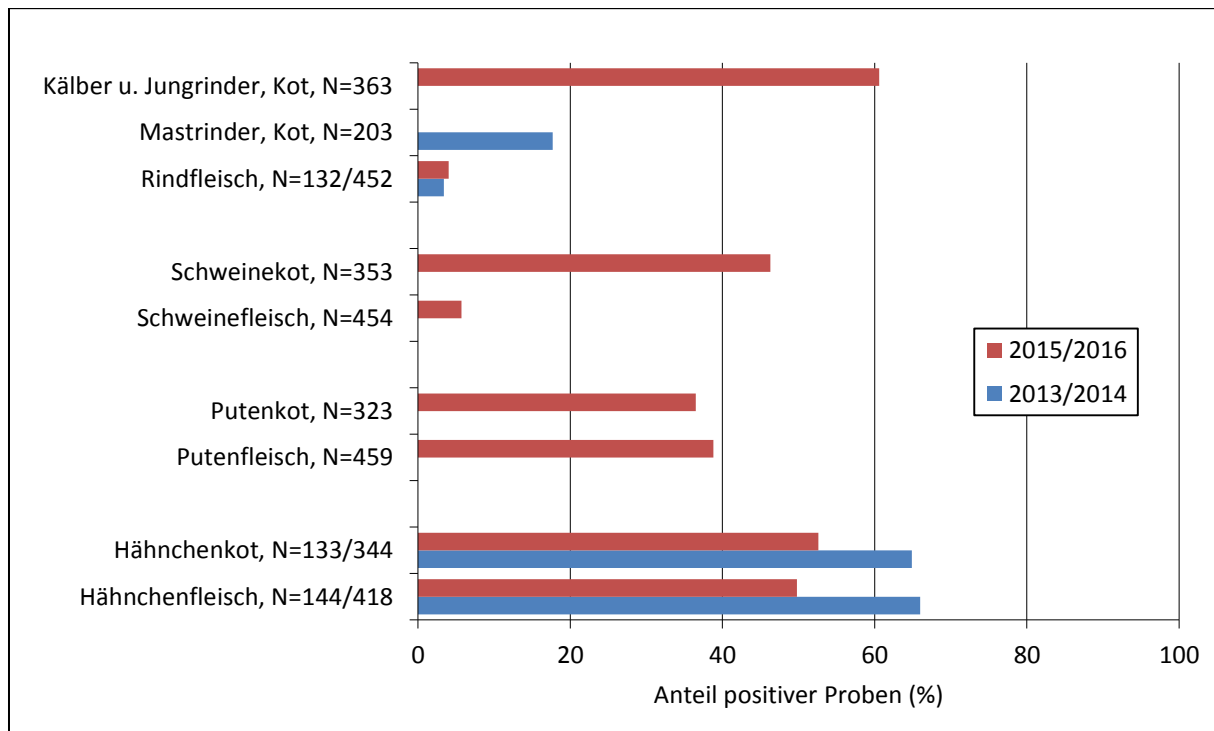
Abbildung 19: Nachweis Cephalosporin-resistenter E. coli mit selektiven Nachweisverfahren in verschiedenen Lebensmittelketten seit 2013 im Zoonosen-Monitoring
