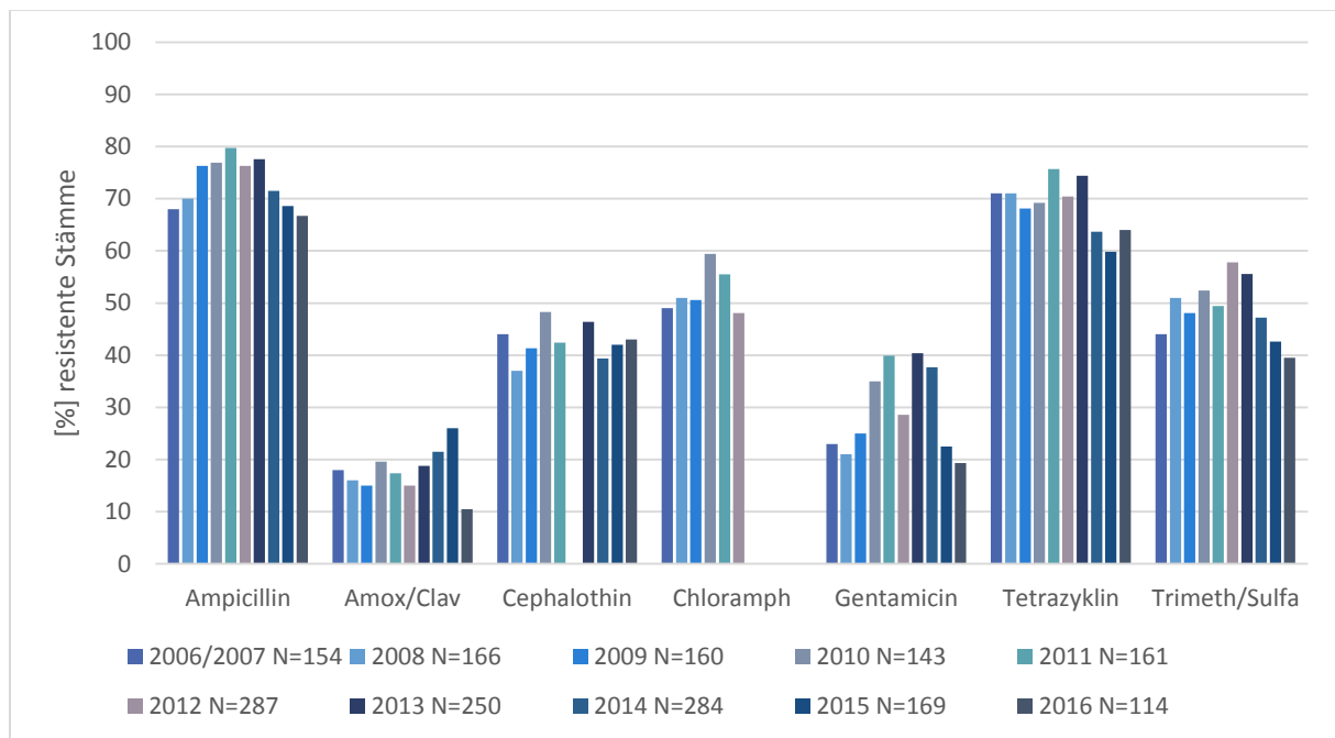
Abbildung 15: Vergleich der Resistenzraten gegenüber antimikrobiellen Substanzen von E. coli isoliert an Enteritis erkrankten Kälbern (Untersuchungszeitraum 2006/2007-2016). 2012 wurde Cephalothin nicht untersucht, Chloramphenicol wurde nur bis 2012 untersucht
