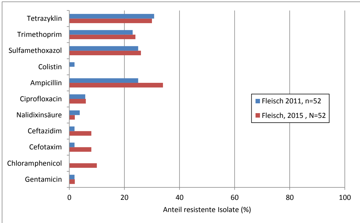
Abbildung 9: Vergleich der Resistenz von E. coli von Schweinefleisch aus den Jahren 2011 und 2015 (jeweils Zoonosen-Monitoring). Bewertung gemäß Durchführungsbeschluss 2013/652/EU.
