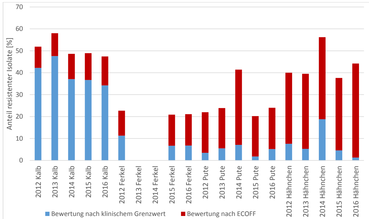
Abbildung 23: Anteil Ciprofloxacin-resistenter E. coli Isolate bei verschiedenen Tierarten, klinische Isolate 2012-2015 mit minimaler Hemmkonzentration über 0,06 mg/l (ECOFF) bzw. 0,5 mg/l (klinischer Breakpoint nach EUCAST), Isolate vom Schwein 2013 und 2014 nicht untersucht.
