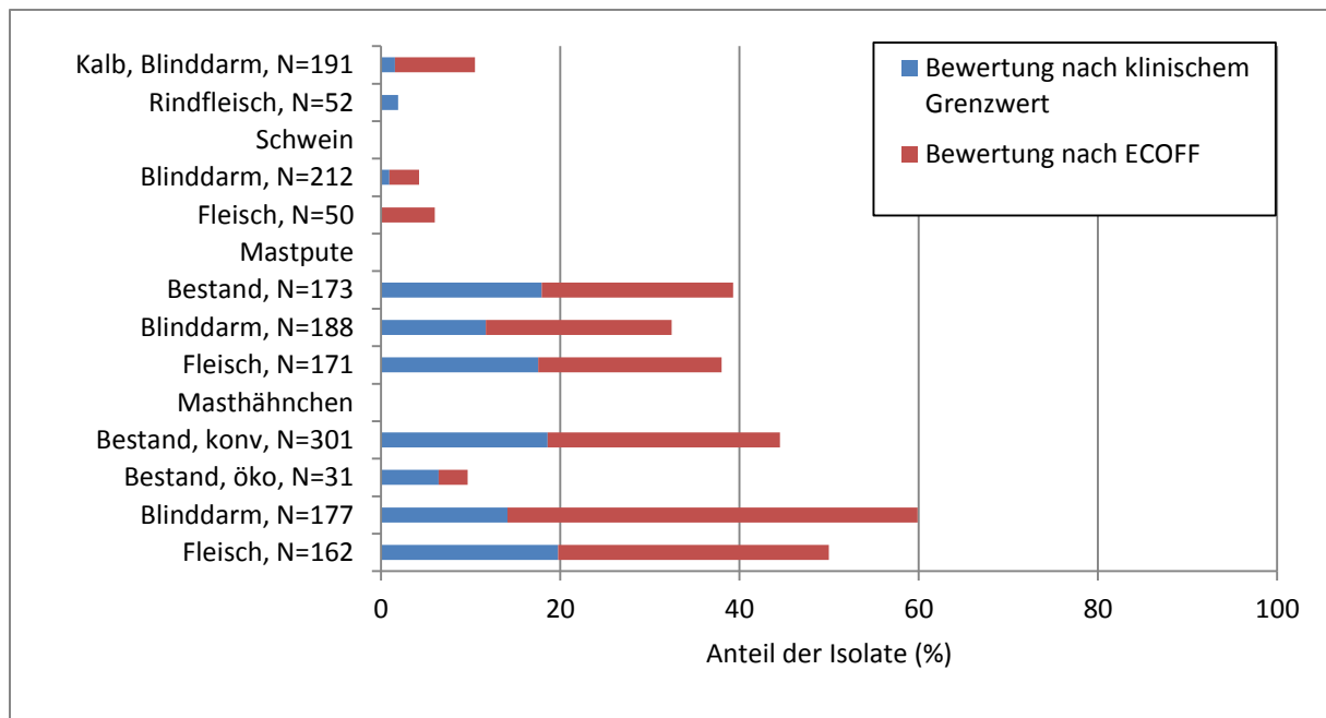
Abbildung 21: Anteil Ciprofloxacin-resistenter E. coli Isolate in den verschiedenen Lebensmittelketten 2015/16 . Bewertung nach klinischem Grenzwert ( >0,5 mg/l) und epidemiologischem cut-off Wert (ECOFF, \leq 0,06 mg/l)
