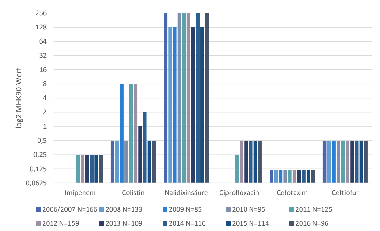
Abbildung 8: Vergleich der MHK 90 -Daten gegenüber antimikrobiellen Substanzen von E. coli , isoliert aus erkrankten Puten (Untersuchungszeitraum 2006/2007-2016, Ciprofloxacin und Imipenem seit 2012 untersucht)
