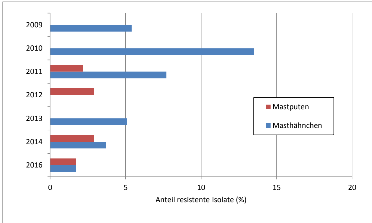
Abbildung 17: Anteil Cephalosporin-resistenter E. coli aus nicht selektiver Anzucht bei Masthähnchen und Mastputen 2009-2016 (Puten 2009, 2010 und 2013 nicht untersucht, Hähnchen 2012 nicht untersucht). Bewertung gemäß Durchführungsbeschluss 2013/652/EU.
